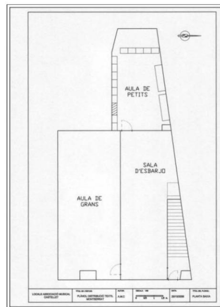
Planta baixa
